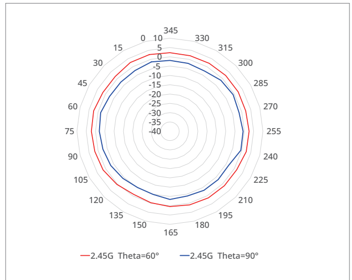
2.4 GHz (ANT1, 2, 3, 4)
