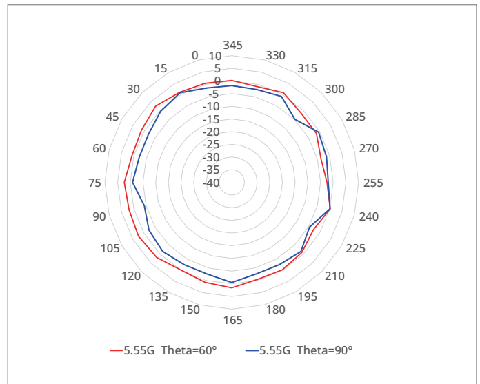
5.5 GHz (ANT1, 2, 3, 4)
